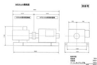
大型 MG 実験装置-鉛蓄電池再生技術室
