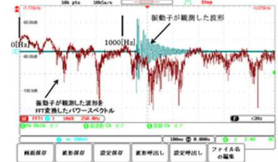
図 3 ひび割れ有のヒューム管のスペクトル
