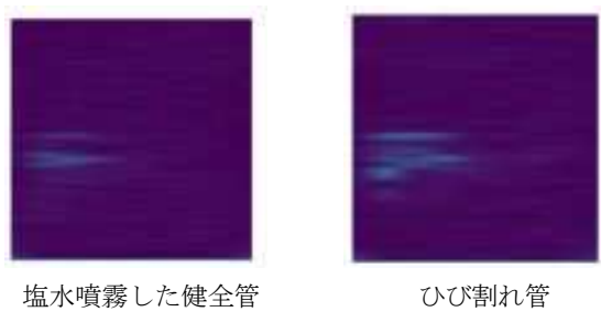
図 4 塩水噴霧した健全管とひび割れ管の STFT 画像
