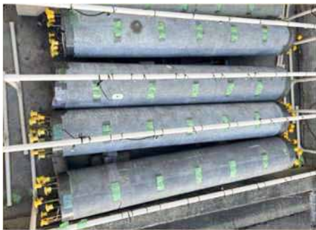
写真 2 2m電柱の塩水噴霧の状況
