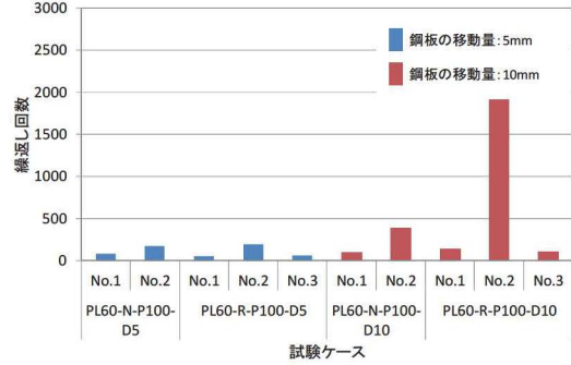
(b) 鋼板の移動量による違い
