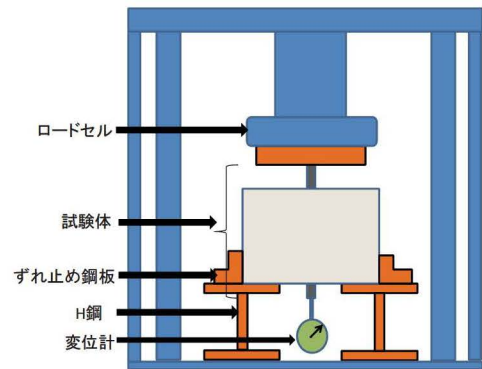
図-2 試験方法
