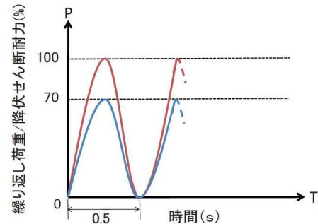
図-3 繰返し荷重の種類
