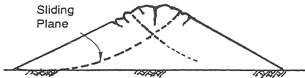
(d) Cracking and Sliding in Earth Dam
