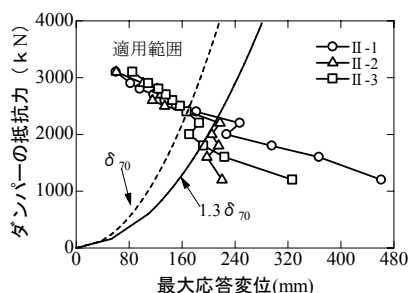
図-13 パネルダンパーの平均せん断ひずみの照査(II種地盤)
