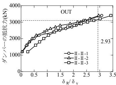
図-12 橋脚の残留変位の照査(II種地盤)
