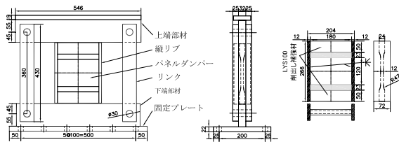
図-1 供試体寸法
