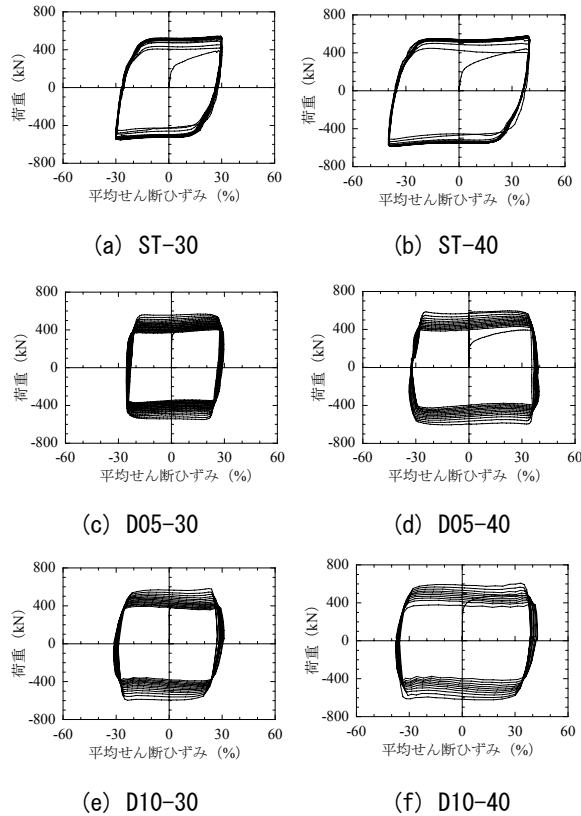
図-3 履歴曲線(平均せん断ひずみ 30%, 40%の例)
