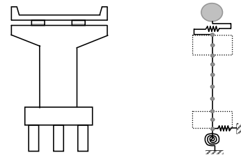
(a) 橋梁の概略図 (b) 橋梁のモデル
