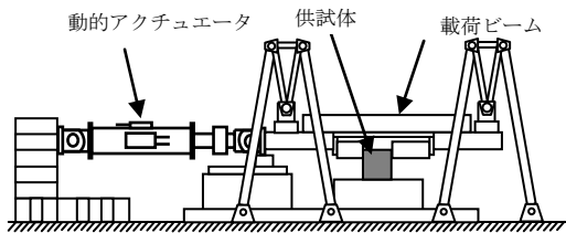
図-2 実験装置
