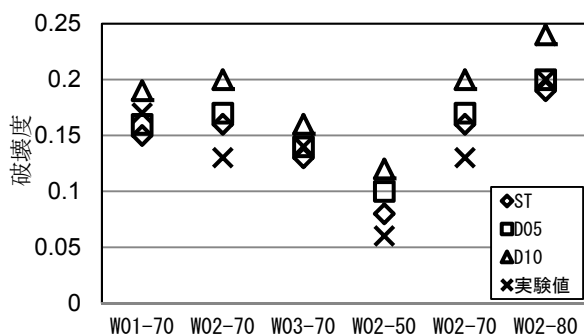
図-21 破壊度の検討
