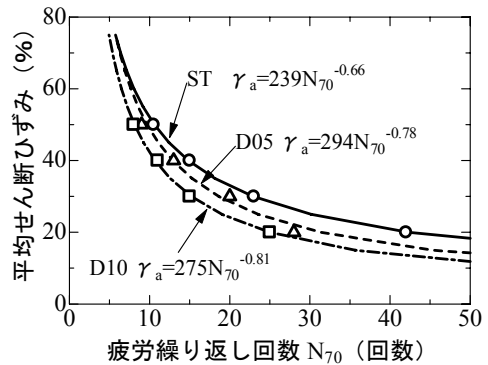
図-6 疲労曲線
