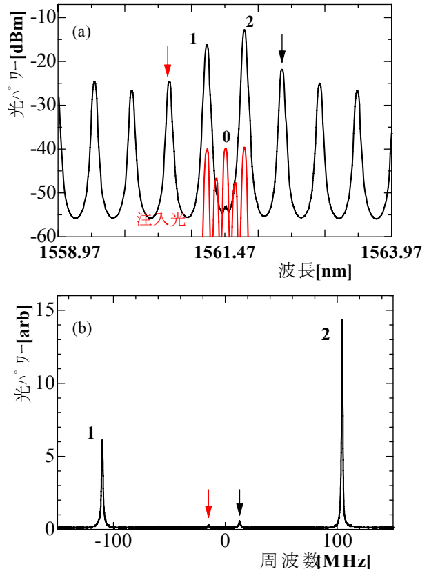
図 4.3 共振器長 600μm の F-P LD (搬送波抑圧あり)
